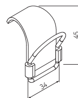
BAND HANGER 밴드걸이
