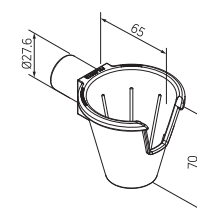
TOOL HOLDER - B 공구걸이캡
