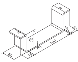
FORKLIFT HOOK 지게차포크 이탈방지 금구
