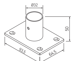
STANCHION MOUNT 바닥고정금구
