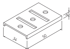
HANDLE FIXING-A, 손잡이 고정금구-A
