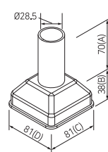
SQUARE CAP 사각종발이
