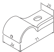
PIPE CLAMP-A, 안장금구-A
