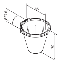
TOOL HOLDER - A 공구걸이캡
